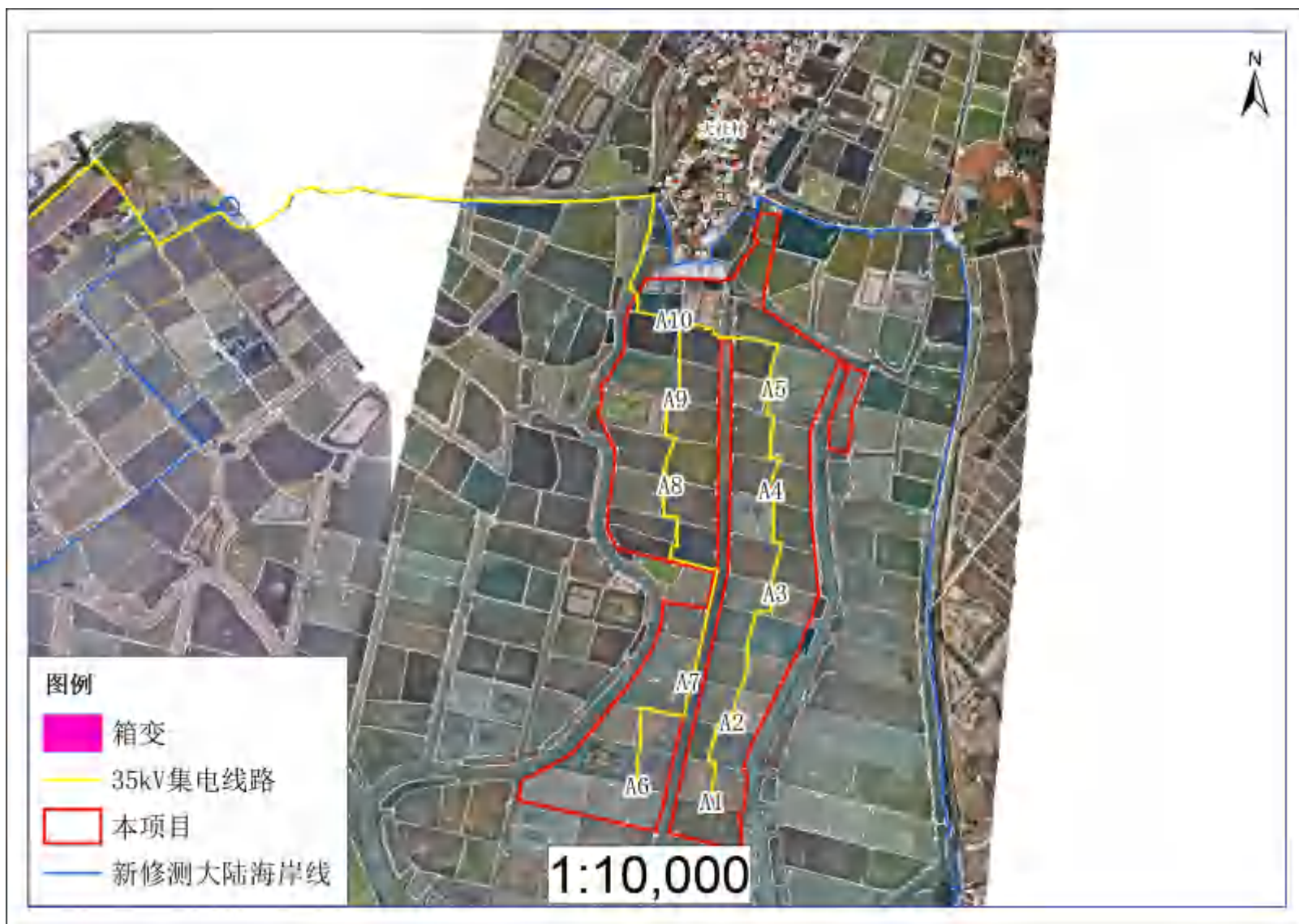
图 4.7-1 箱变与周边居民区的位置关系
