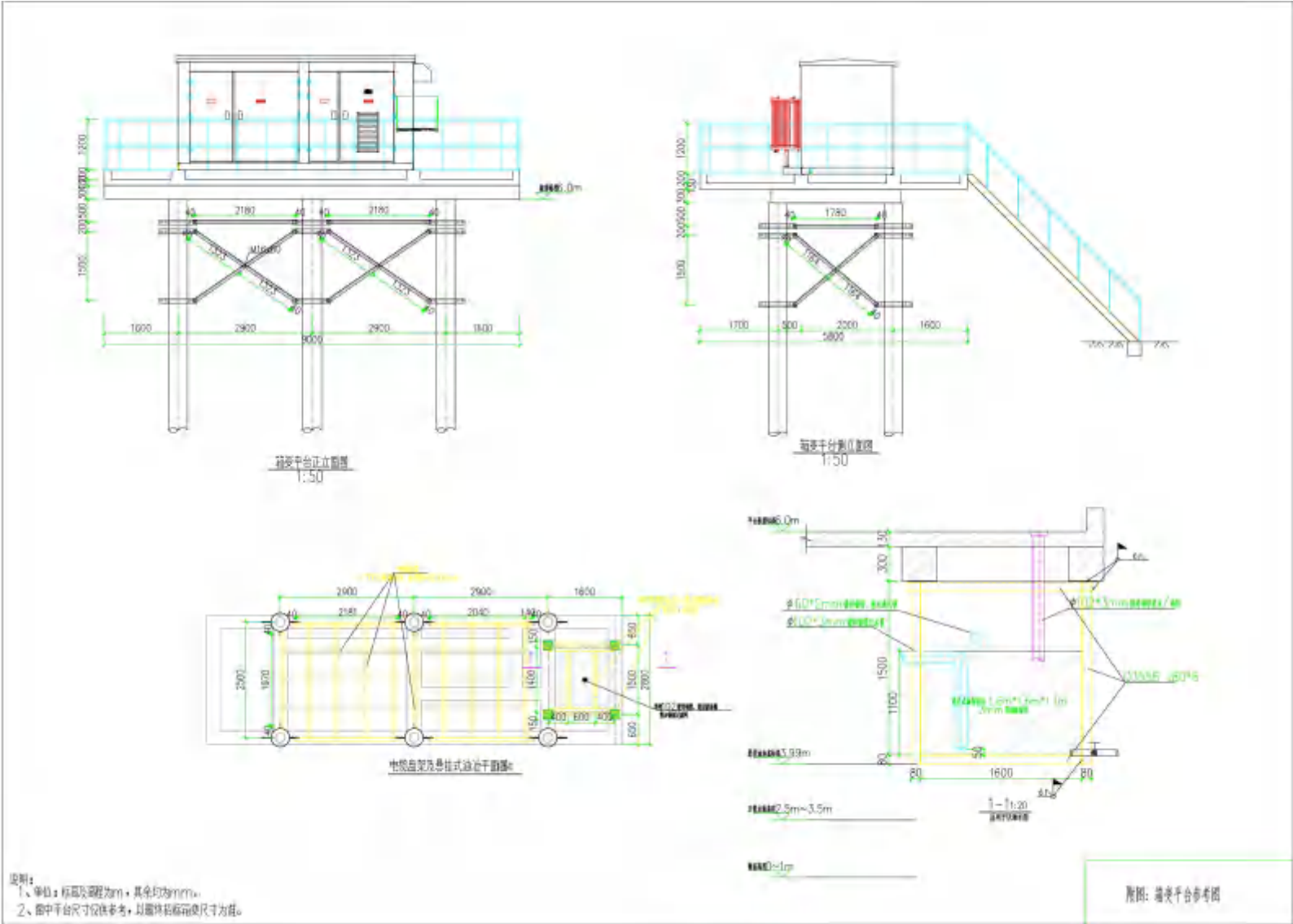
图 2.5-19 事故油池结构图
