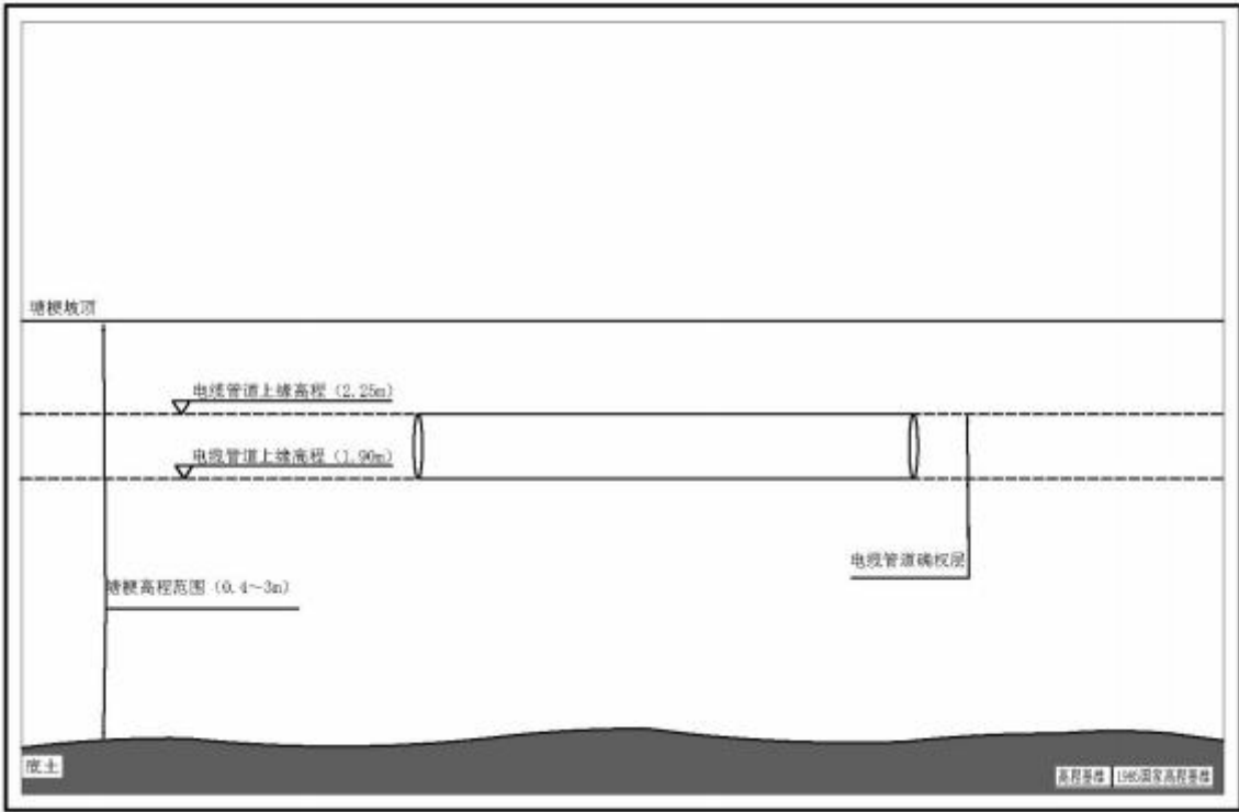
图 2.5-14 电缆沟剖面图
