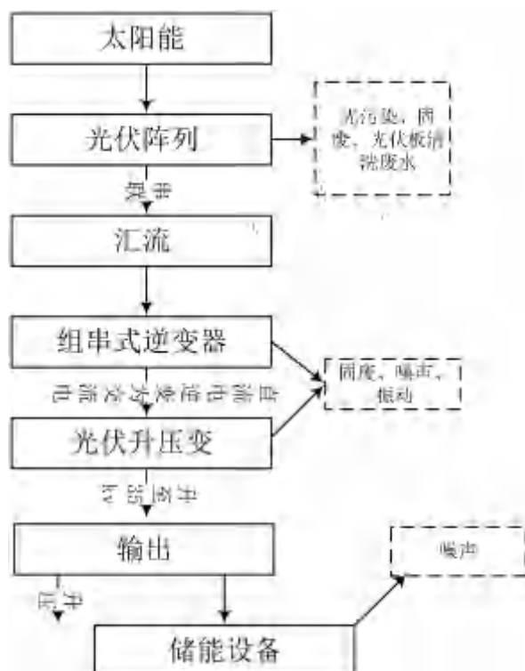
图 2.10-1 本项目运营流程及产污环节示意图
