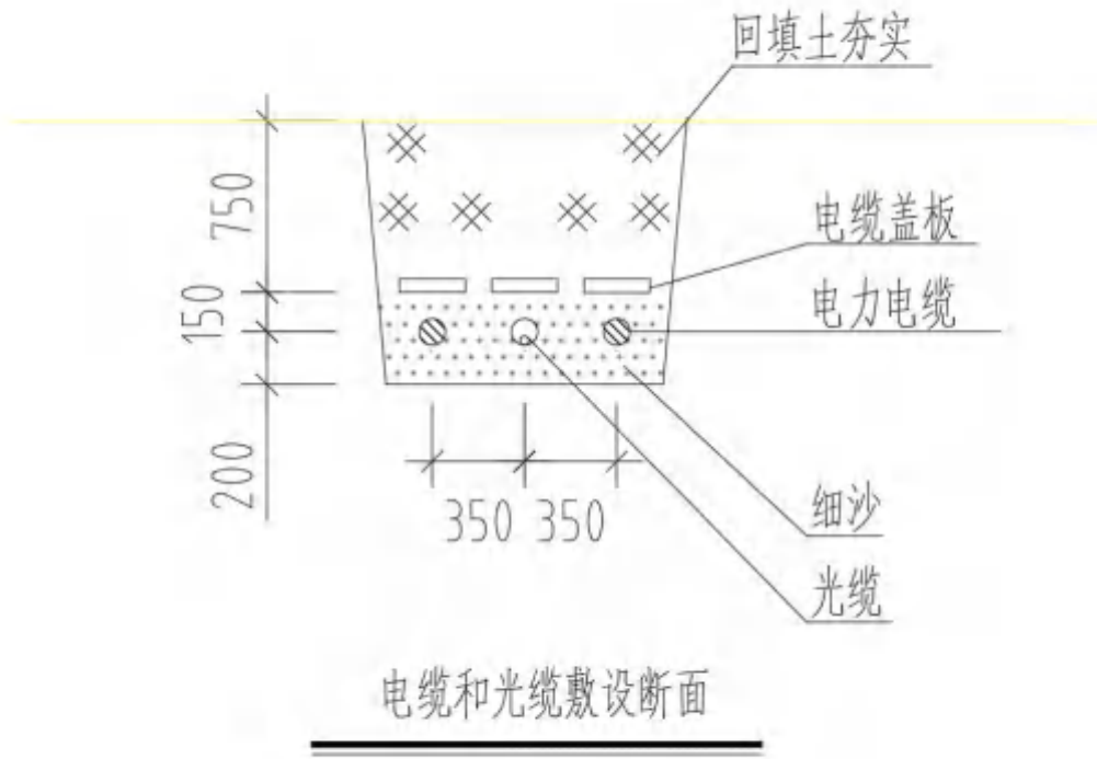
图 2.5-15 埋地电缆断面图
