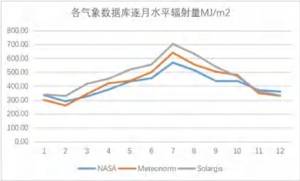
图 3.1-11 各气象数据库逐月水平辐射量对比图 (MJ/m²)
