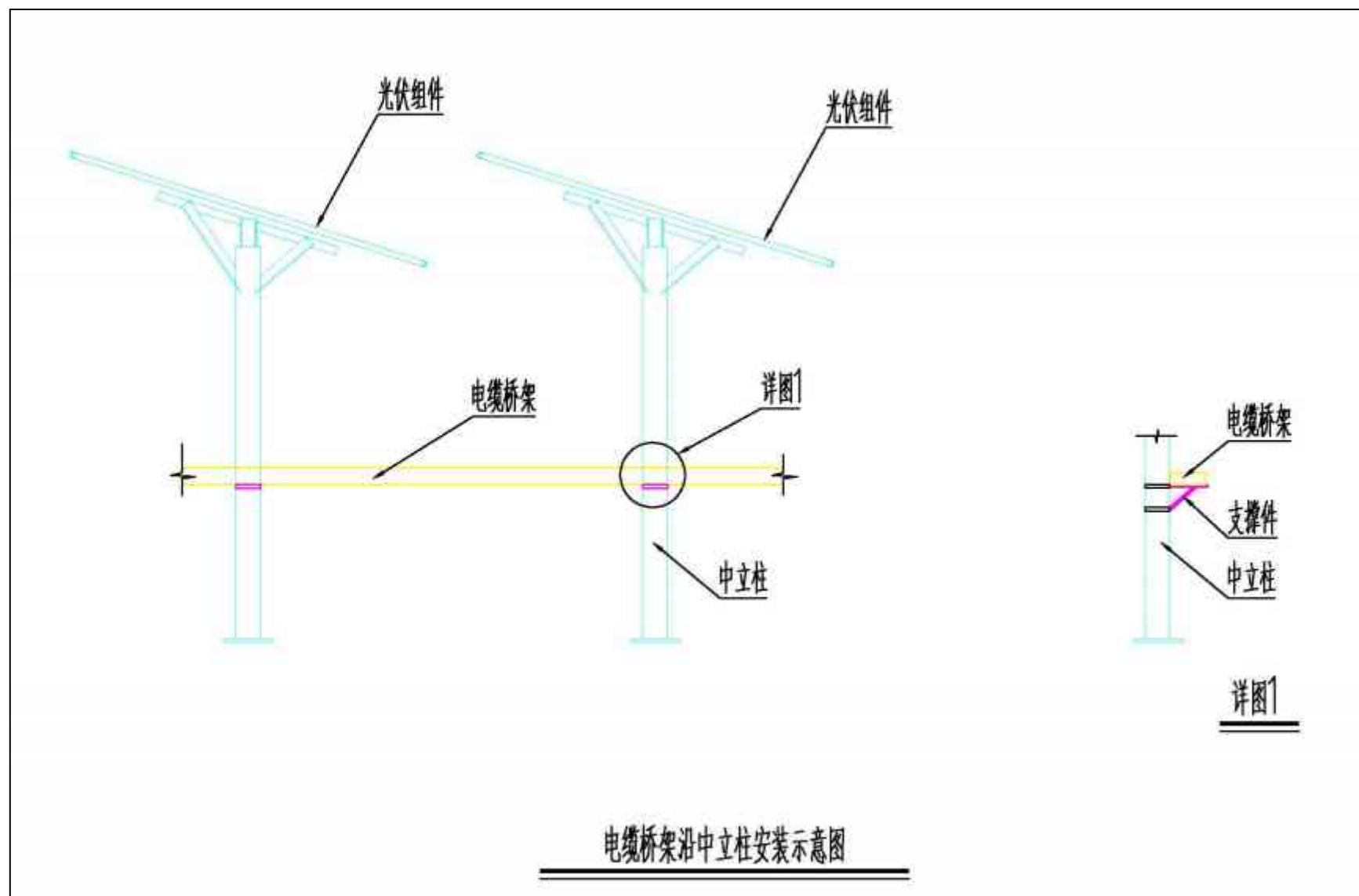
图 2.5-10 电缆桥架安装示意图
