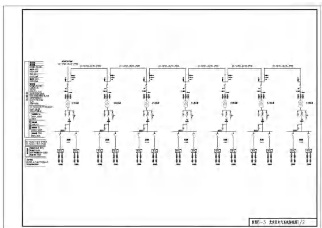
图 2.5-8 光伏配电系统接线示意图
