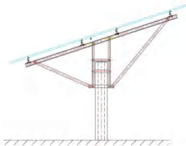
图 2.5-4 固定支架结构示意图
