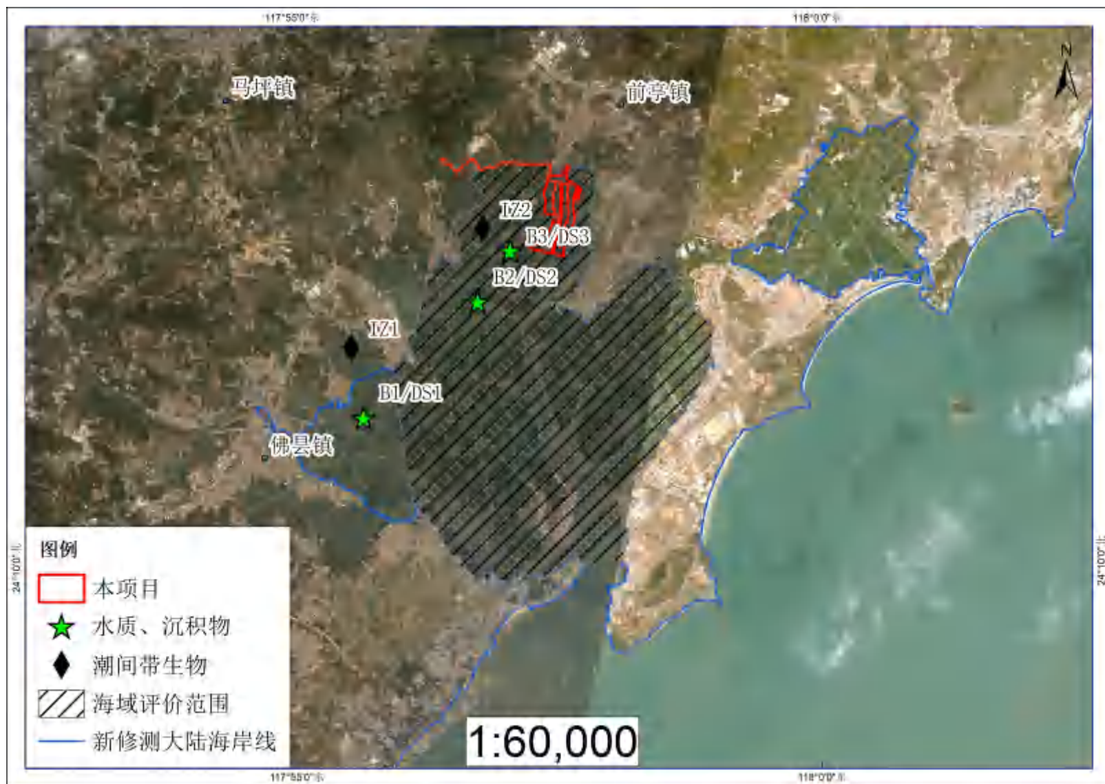
图 3.3-1 海洋生态环境监测站位分布图
