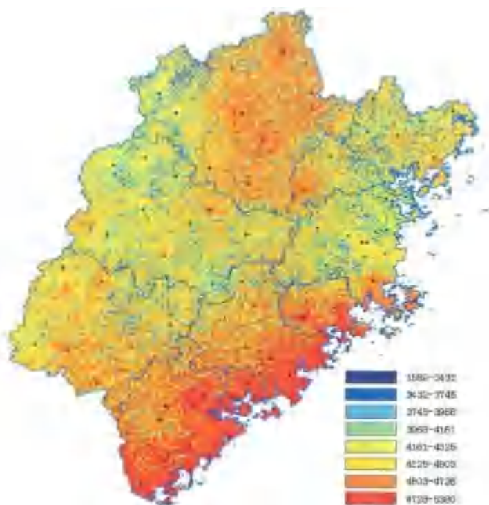
图 3.1-9 福建省年平均年太阳能总辐射分布图 (MJ/m 2 )
