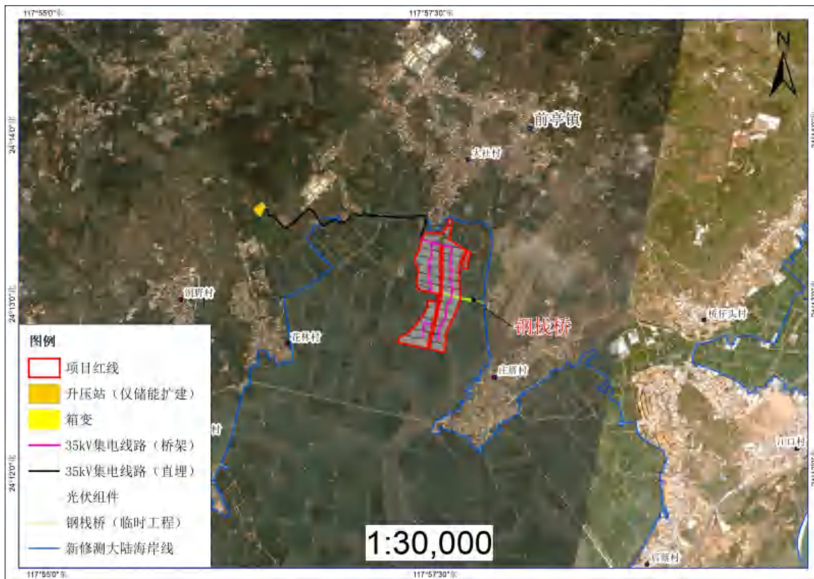
图 2.5-21 临时钢栈桥位置示意图
