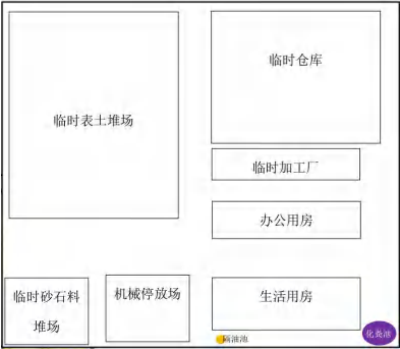
图 2.5-25 本项目依托工程（升压站施工营地）总平面布置图
