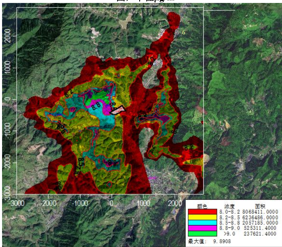
图5 项目新增污染源及拟建污染源正常排放时叠加背景值后 NO 2 年均浓度分布图，单位 \mu\text{g}/\text{m}^3
