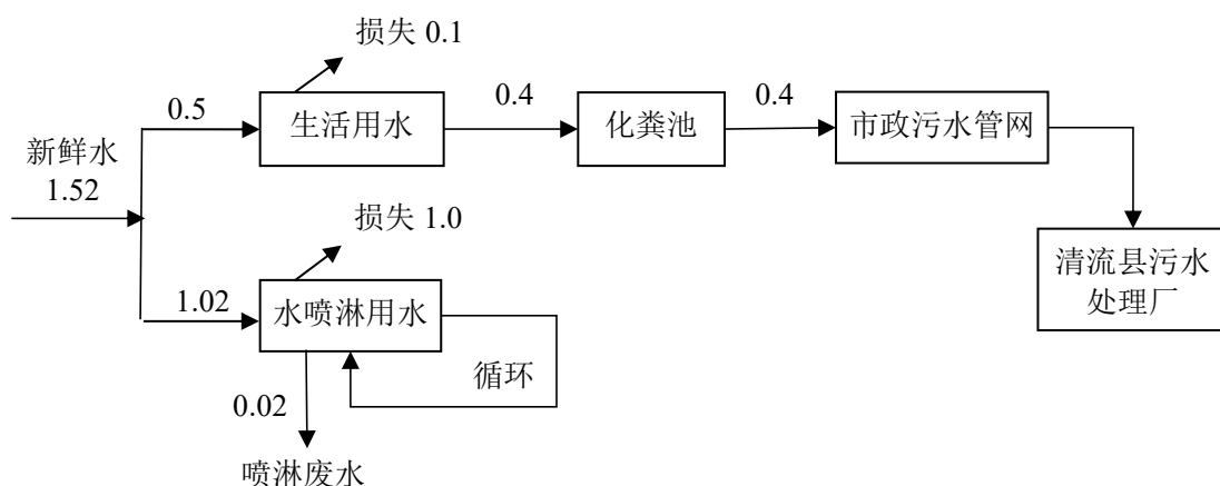
图 2.1-1 项目水平衡图 单位：t/d
