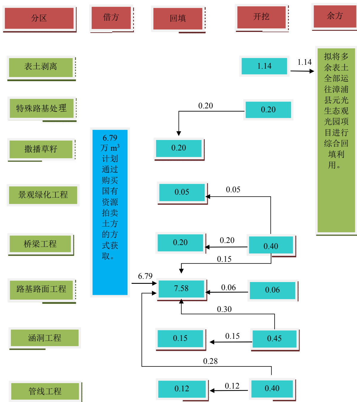
图 2-4 项目土石方流向框图单位：万 m³
