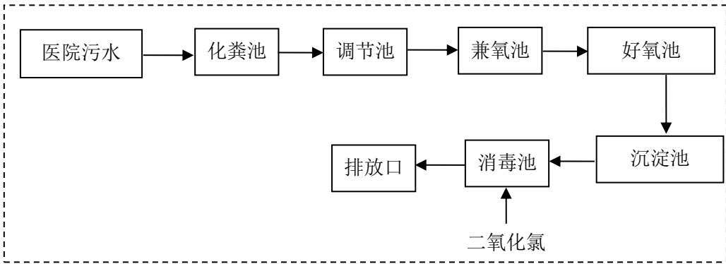
图 5-1 废水处理设施工艺流程图
