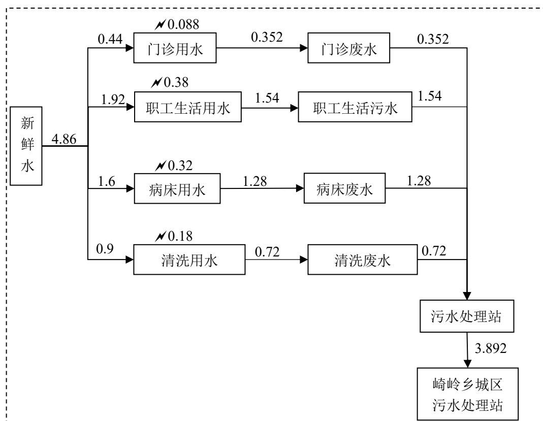
图 3-1 项目水平衡图 单位：t/d
