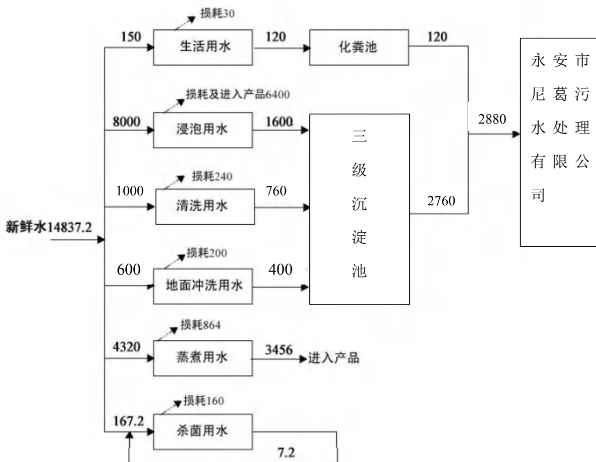
图 2-1 水平衡图
