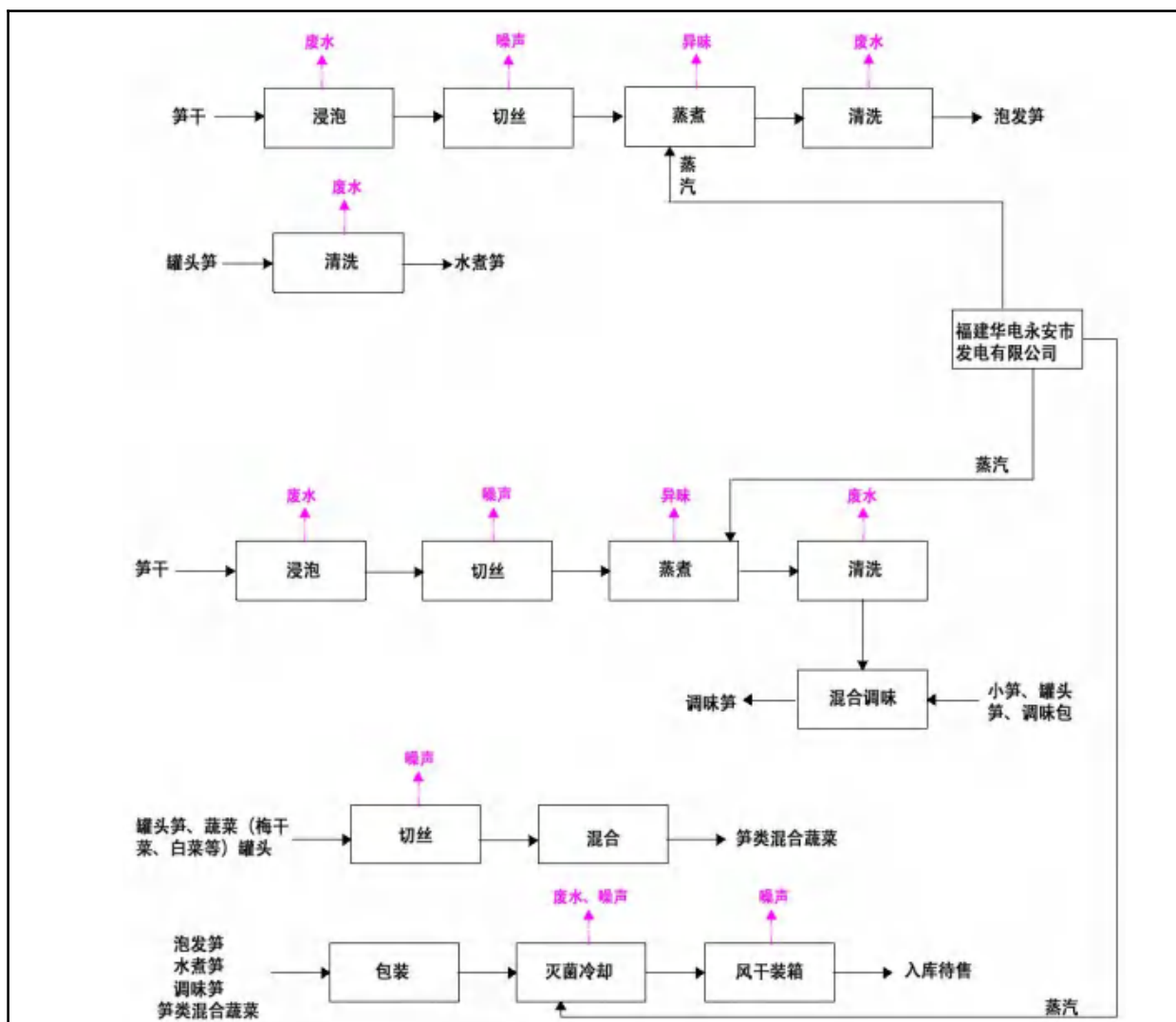
图 2-2 生产工艺流程及产污环节图
