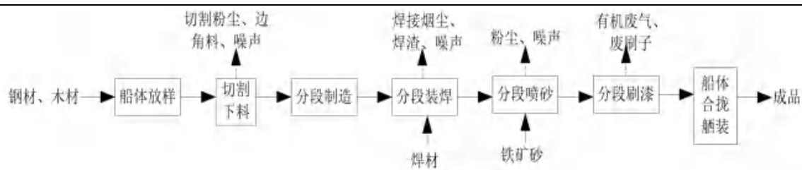
图 3-5 钢质渔船生产工艺流程图
