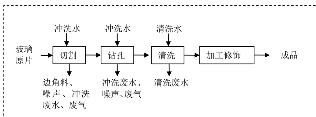
图 2.8-2 一般工艺、包装用品玻璃工艺流程图
