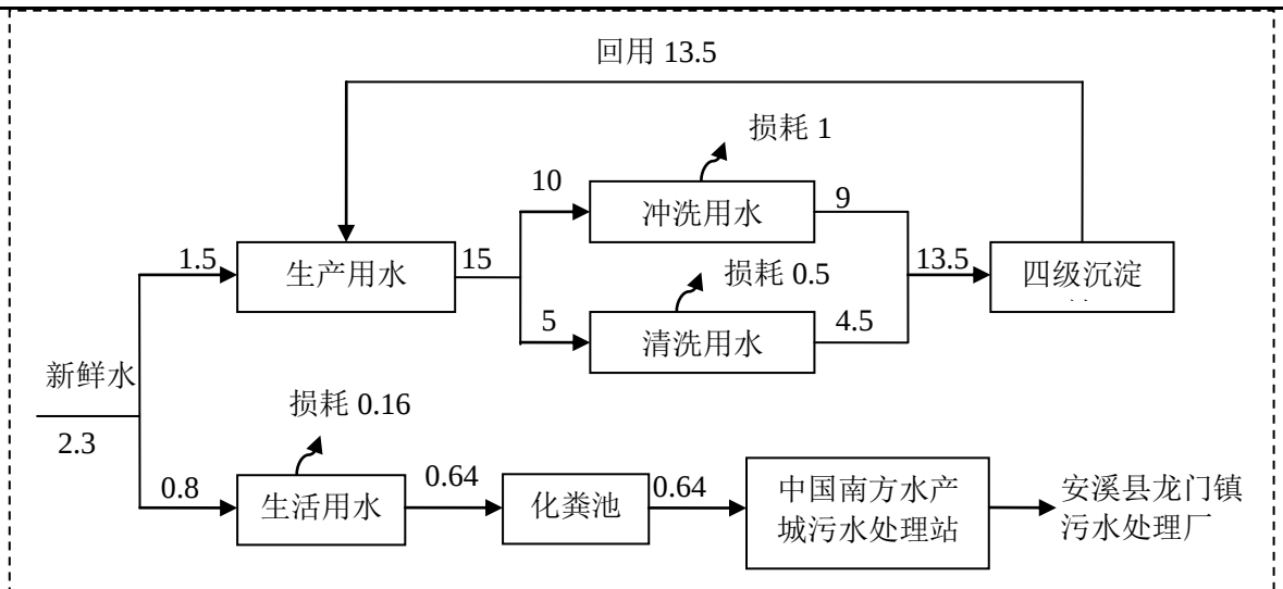
图 4.2-1 项目水平衡图（单位 t/d）
